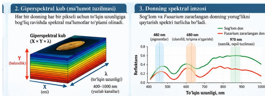
1-rasm. Giperspektral kub va sog'lom hamda Fusarium zararlangan don spektrlarining konseptual farqi (muallif ishlanmasi)
