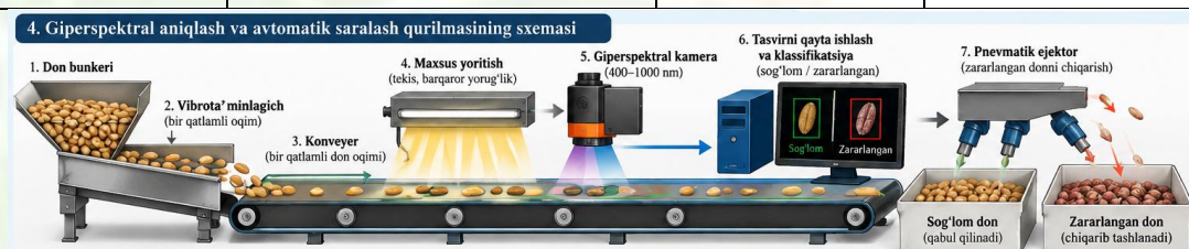
2-rasm. Fusarium zararlangan bug'doy donini aniqlash va pnevmatik ajratishning konseptual texnologik sxemasi (muallif ishlanmasi)
